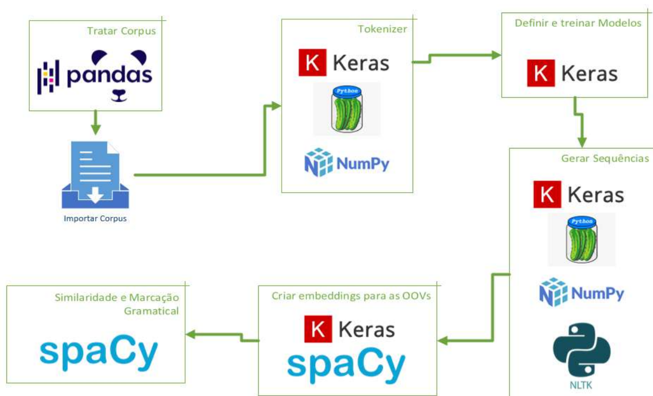
Figura 6 – Fluxo da implementação do experimento
