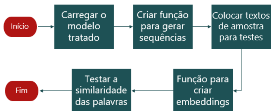
Figura 8 – Fluxo para a predição de Embeddings
