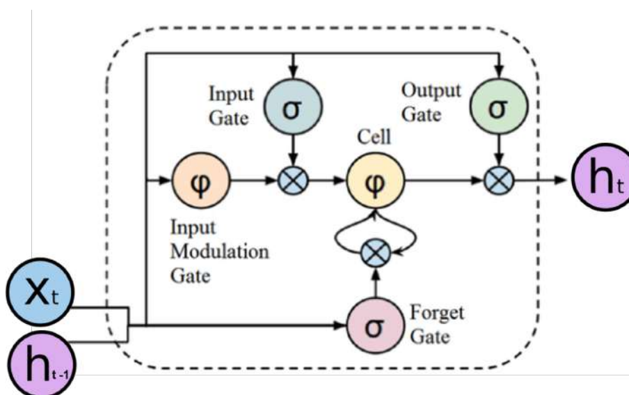
Figura 3 – Arquitetura de uma LSTM
