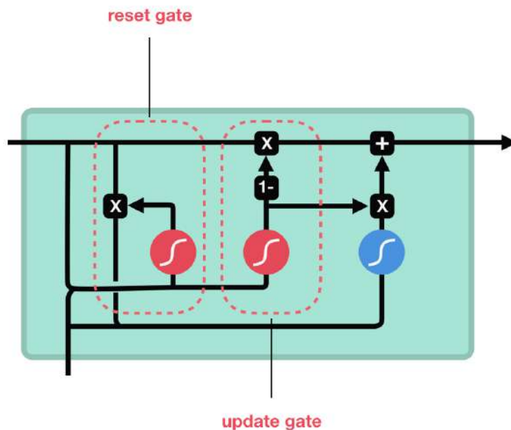
Figura 4 – Arquitetura de uma GRU
