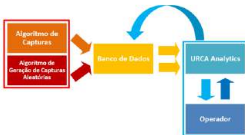
Figura 14: Esquema de integração das aplicações até URCA Analytics
