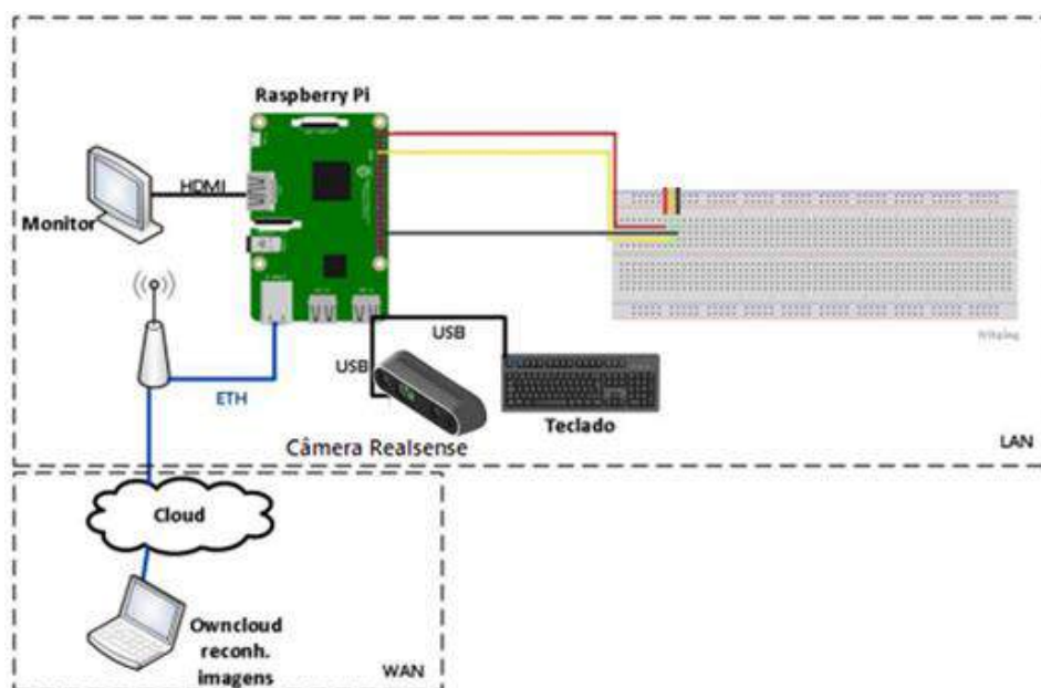
Figura 8: Projeto para a prova de conceito
