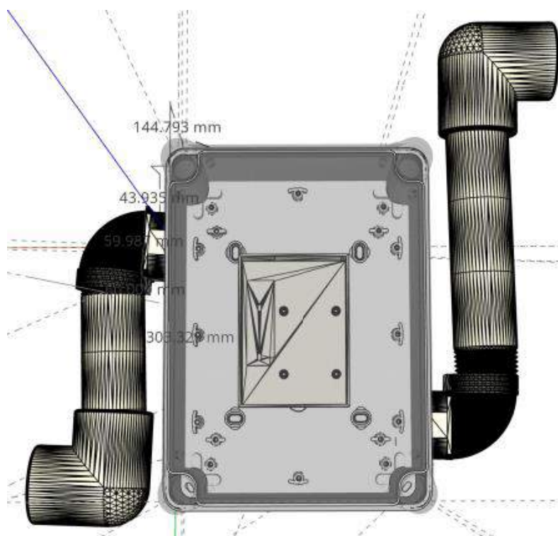
Figura 24: Modelagem 3D do encapsulamento mecânico para o ambiente outdoor
