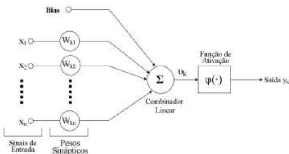
Figura 3: Representação de um neurônio Artificial
