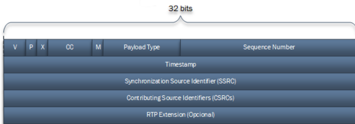
Figura 6: Cabeçalho RTP. Fonte: Autor.
