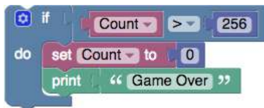
Figura 6 - Trecho de programa em linguagem visual.
