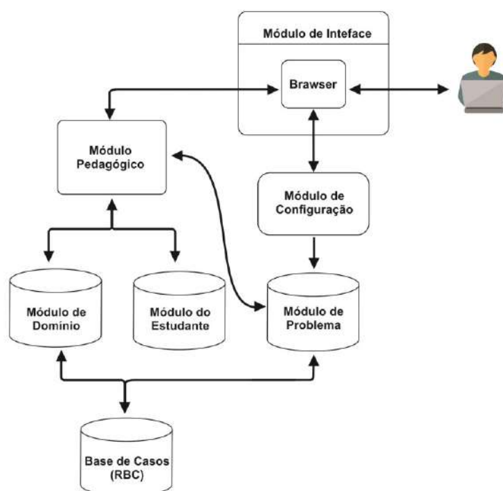
Figura 21 - Arquitetura Geral do STI BLOP.
