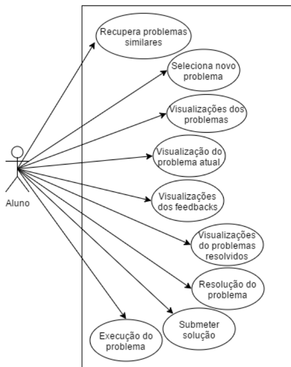
Figura 23 - Diagramas de casos de usos Aluno.
