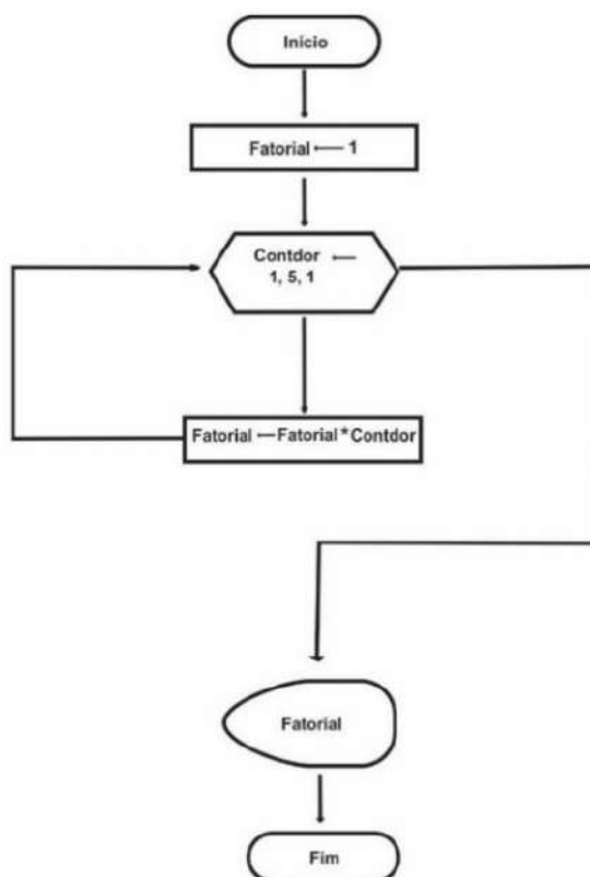
Figura 3 - Fluxograma: cálculo do fatorial de N.
