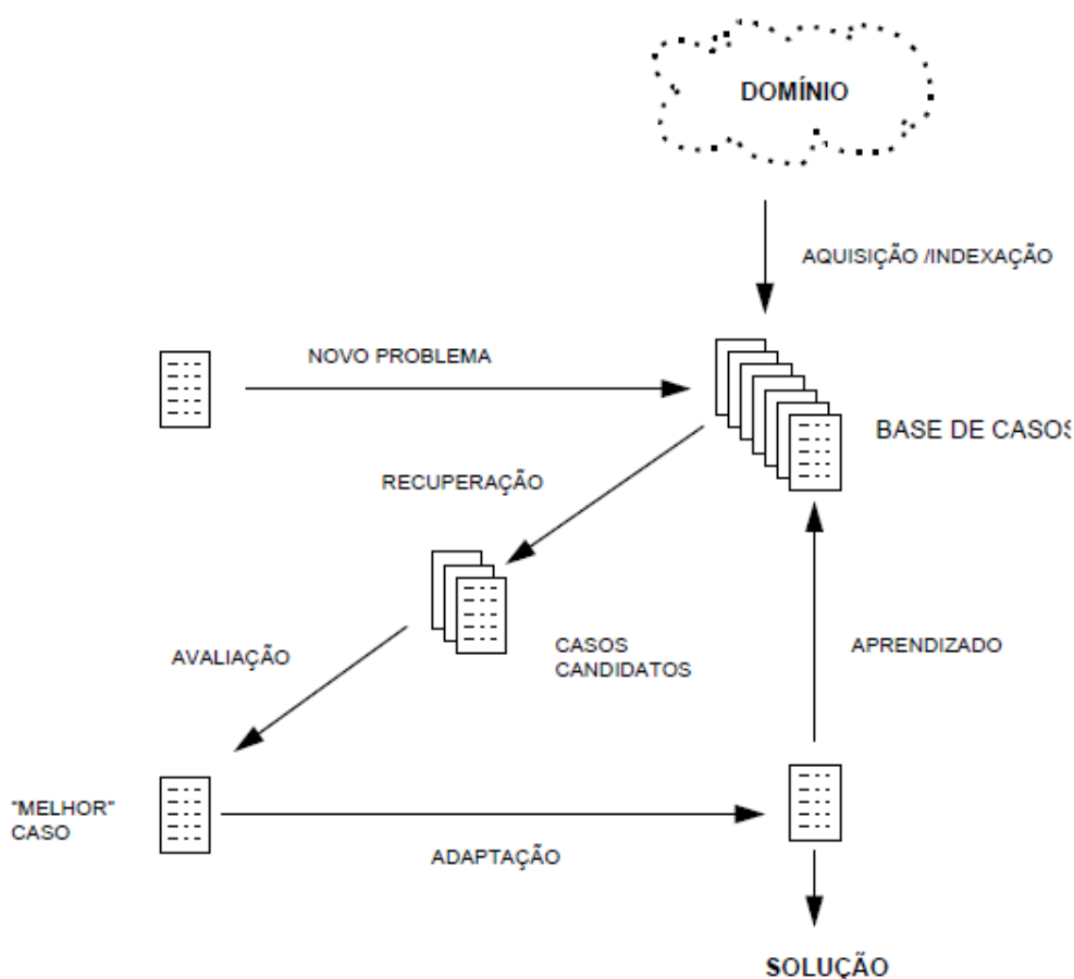
Figura 16 - Ciclo de solução de problema de um sistema CBR (WANGENHEIM; WANGENHEIM & RATEKE, 2013).
