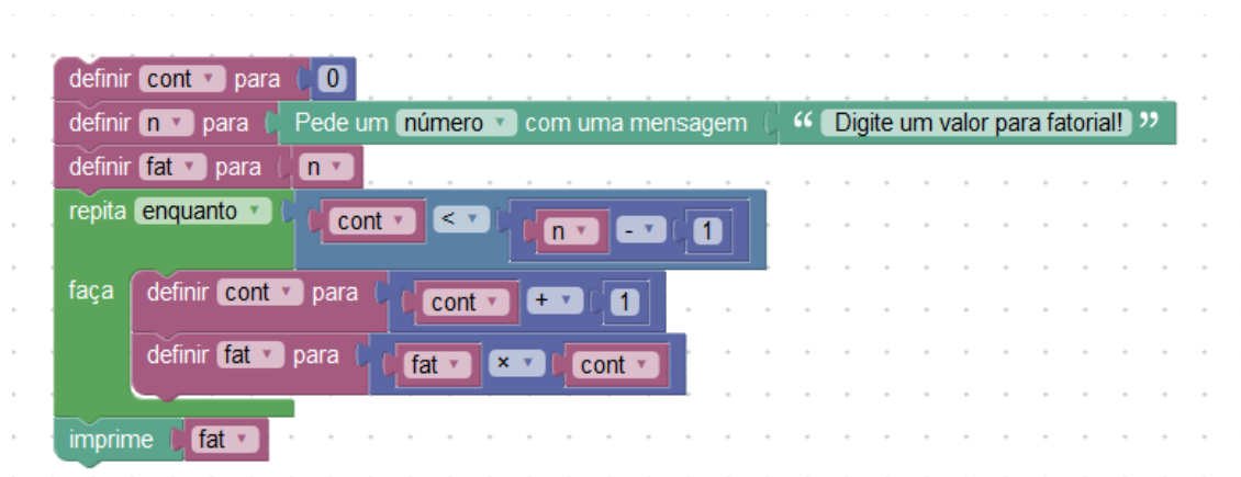
Figura 5 - Linguagem visual em blocos fatorial de N.
