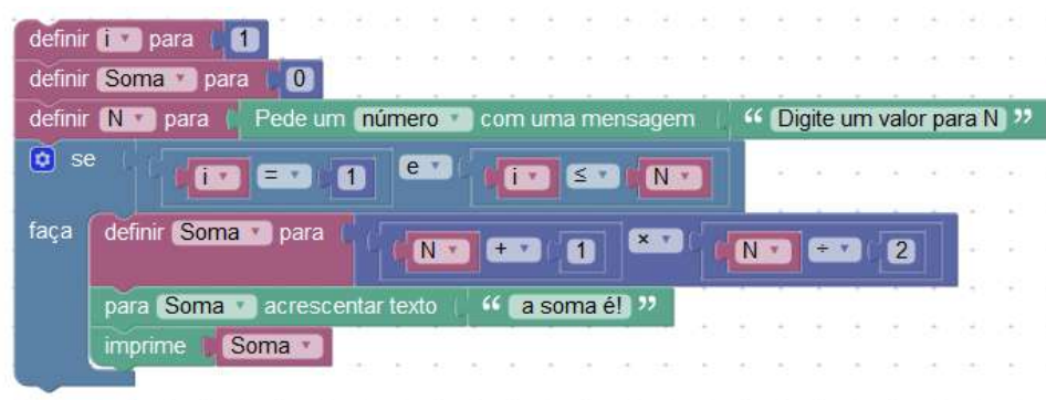
Figura 19 - Linguagem visual problema soma.
