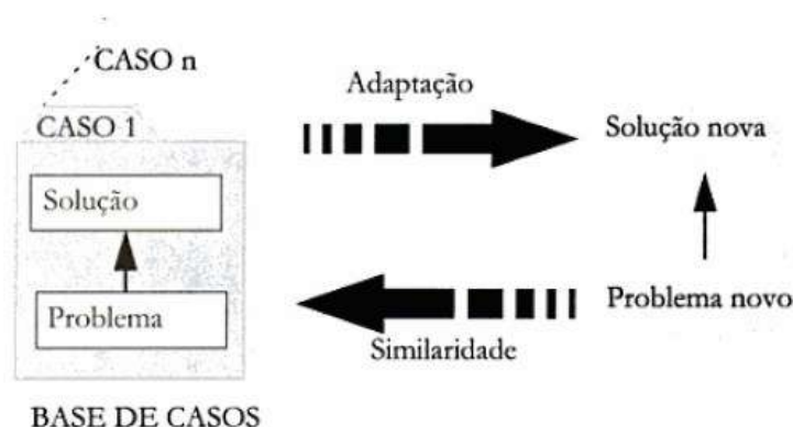
Figura 15 - Modelo do Raciocínio Baseado em Casos (WANGENHEIM; WANGENHEIM & RATEKE, 2013).
