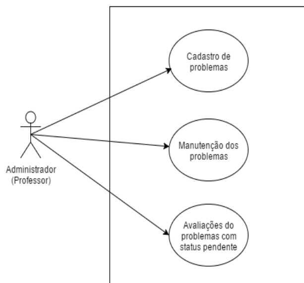
Figura 22 - diagramas de casos de usos Administrador/Professor.
