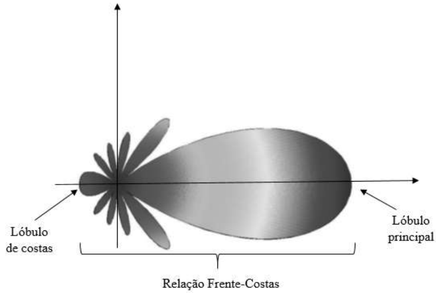
Figura 2.8 – Relação frente-costas (Fonte: Autor).
