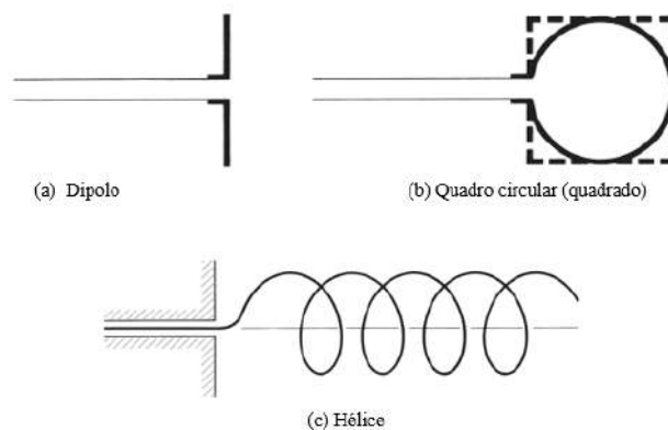
Figura 2.1 – Ilustração de antenas filamentos (BALANIS, 2016).
