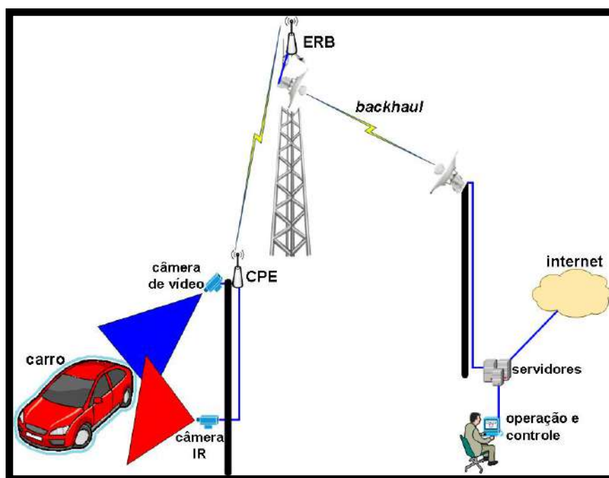
Figura 10. Topologia URCA
